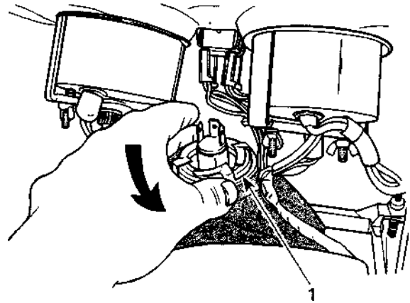
1. Ламподержатель
