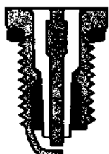
Тип удлиненного изолятора
